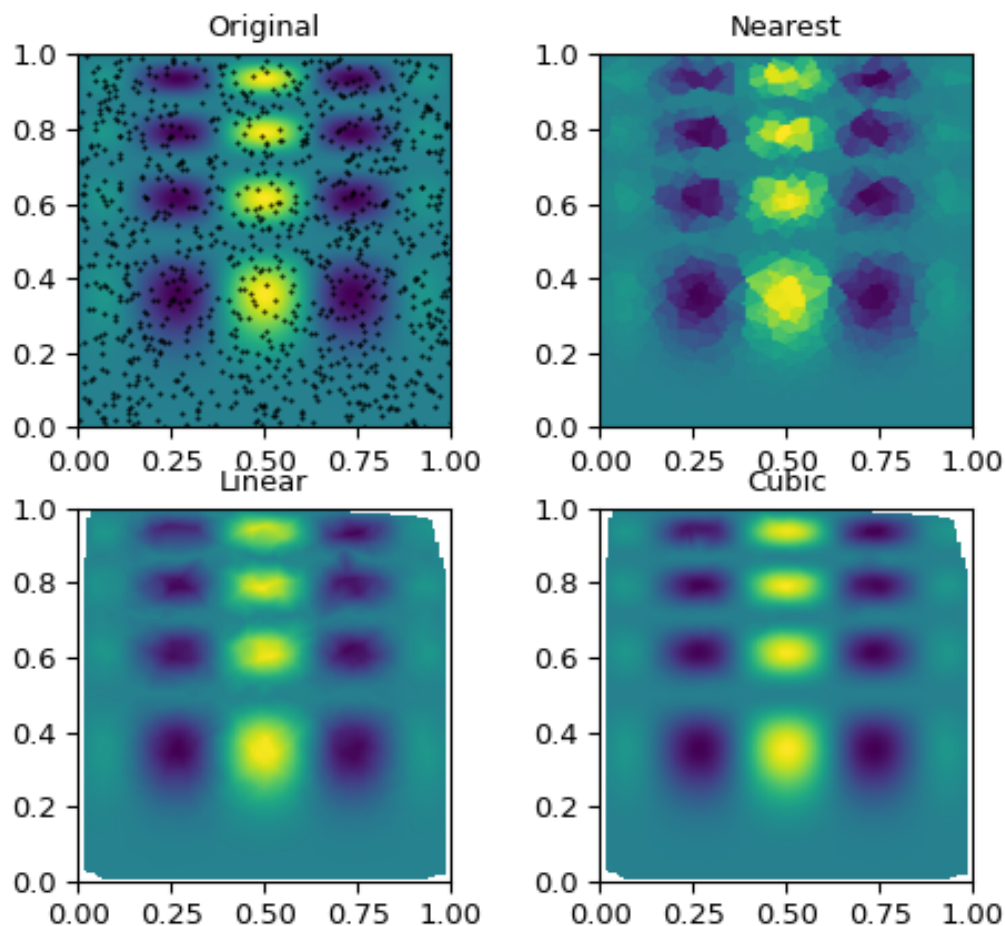
FIGURE 24 – Différents Types d'Interpolationsource. Source : SciPy Documentation
